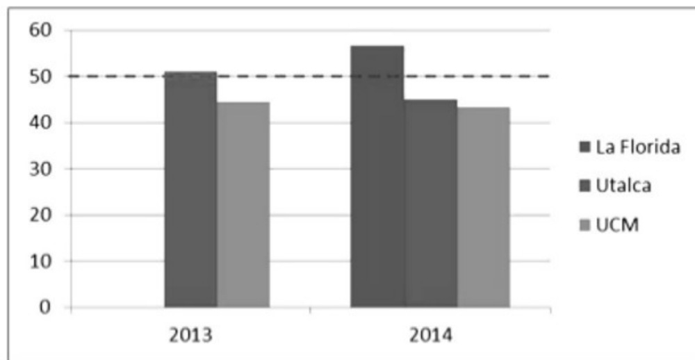
Figura 7. Concentraciones anuales MP10
