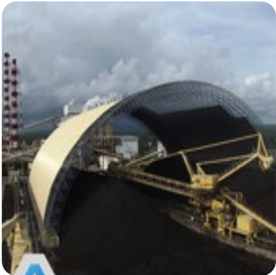
Almacenamiento tipo Hangar para el almacenamiento de carbón, China.
