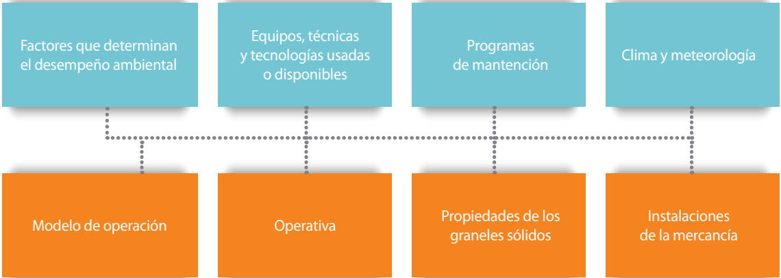
Figura 1.3. Esquema de Factores que determinan el desempeño ambiental en instalaciones que manipulan Graneles Sólidos
