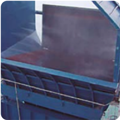
Boca de tolva apantallada con atomizadores de agua de alta presión
