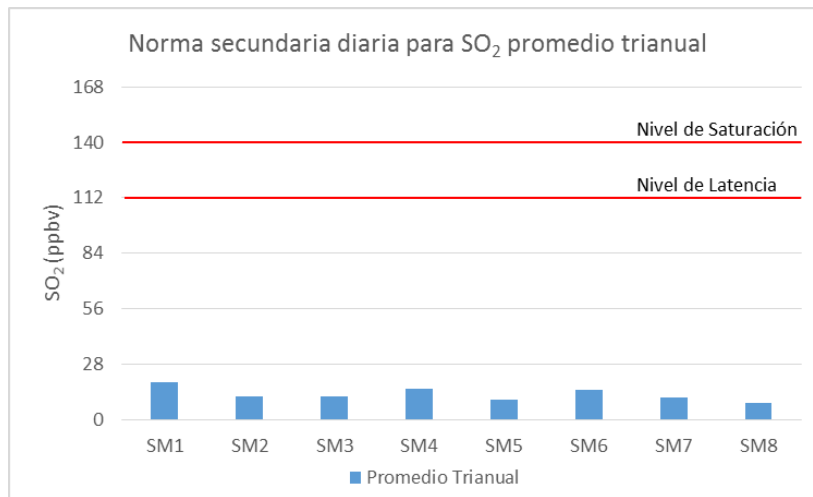
Gráfico 8 Norma secundaria 24 horas para SO 2 , promedio trianual período 2014 al 2016
