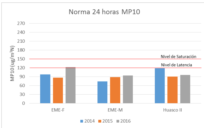
Gráfico 1 Norma 24 horas para MP10, período 2014 al 2016
