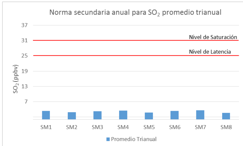
Gráfico 10 Norma secundaria anual para SO 2 , promedio trienal período 2014 al 2016
