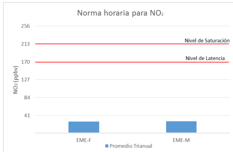
Gráfico 3 Norma 1 hora para NO 2 , promedio trianual período 2014 al 2016
