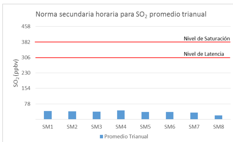
Gráfico 6 Norma secundaria 1 hora para SO 2 , promedio trianual durante el período 2014 - 2016
