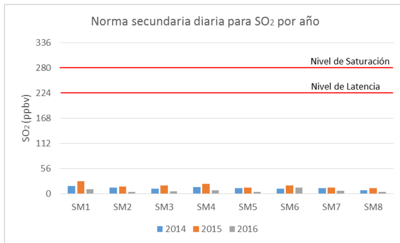
Gráfico 9 Norma secundaria 24 horas para SO 2 , período 2014 al 2016
