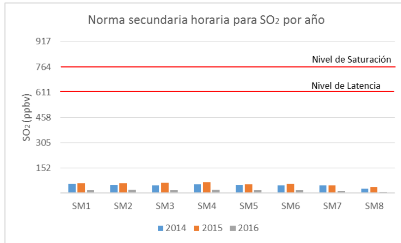
Gráfico 7 Norma secundaria 1 hora para SO 2 , período 2014 al 2016
