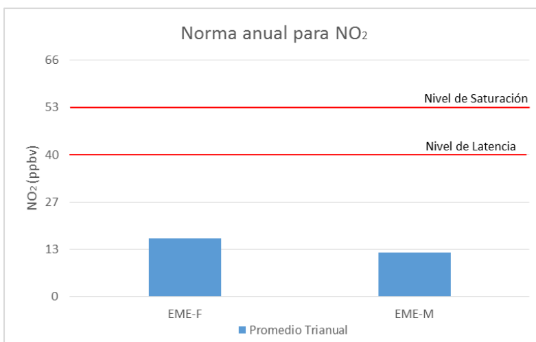
Gráfico 4 Norma anual para NO 2 , promedio trianual periodo 2014 al 2016
