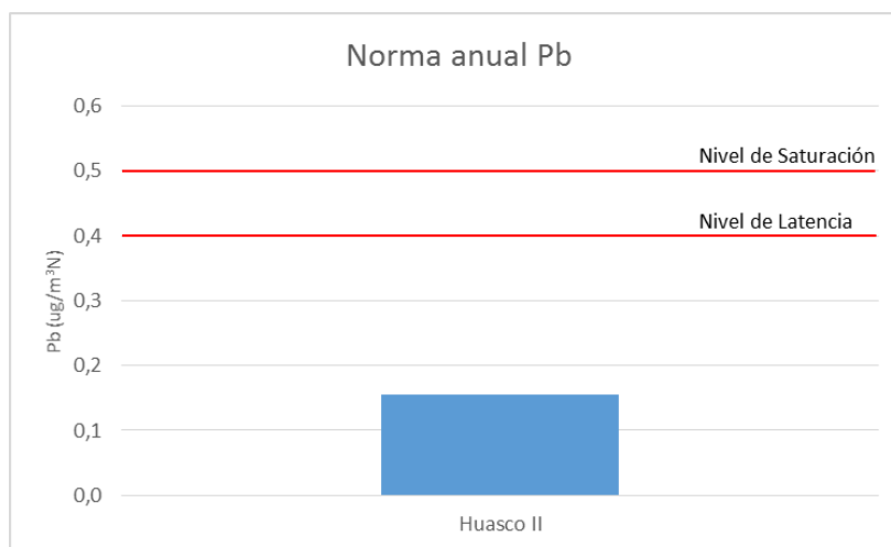
Gráfico 5 Norma anual para Pb, promedio bianual período 2015 al 2016
