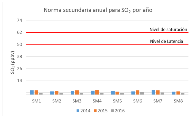
Gráfico 11 Norma secundaria anual para SO 2 , período 2014 al 2016
