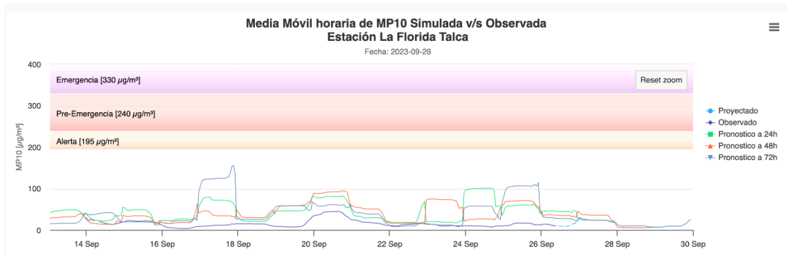
Figura 5. Gráficos de simulación y observación de media móvil 24 h, MP 10 modelo de pronóstico WRF-MMA
