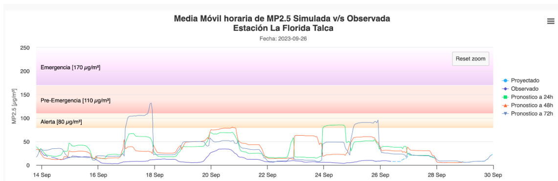
Figura 6. Gráficos de simulación y observación de media móvil 24 h, MP 2,5 modelo de pronóstico WRF-MMA
