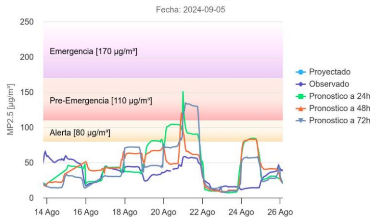
Figura 6. Ejemplo de Gráficos simulación y observación de media móvil 24 h, modelo de pronóstico WRF-MMA
