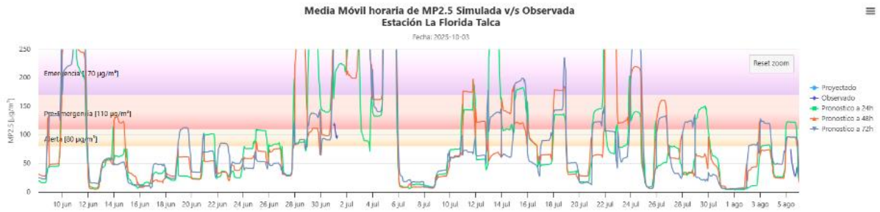
Figura 6. Ejemplo de gráficos de simulación y observación de media móvil 24 h, MP_{2,5} modelo de pronóstico WRF-MMA
