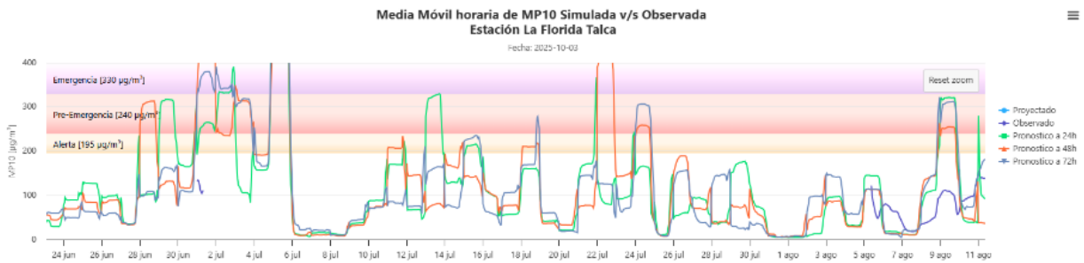
Figura 5. Ejemplo de gráficos de simulación y observación de media móvil 24 h, MP 10 modelo de pronóstico WRF-MMA
